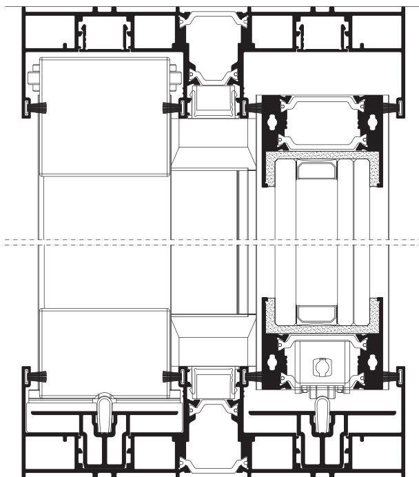
Corte A-A' Section A-A'
