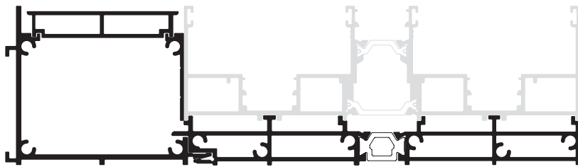
Montagem perfis para caleira Assembly for drainage profile
