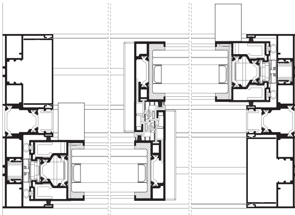
Corte A-A' Section A-A'
